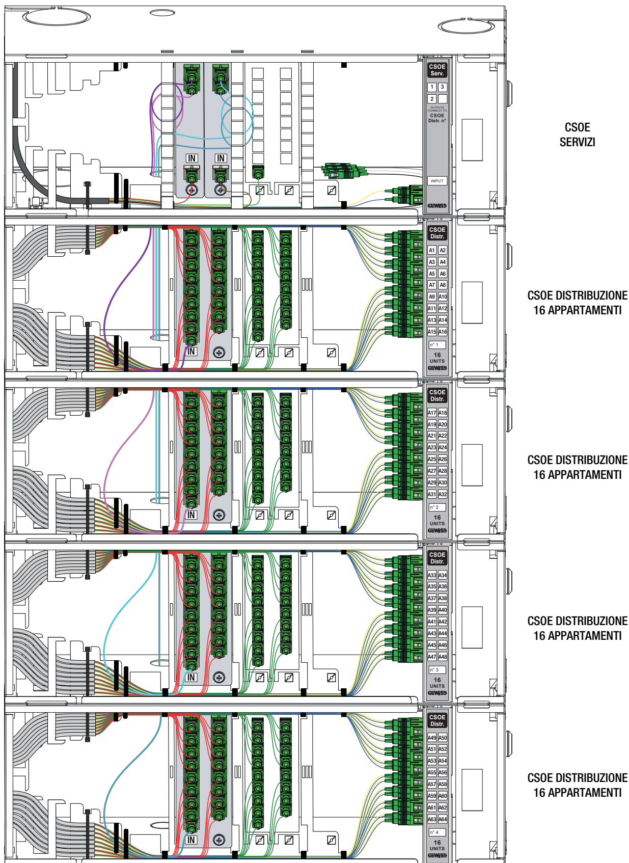
ESEMPIO DI CONFIGURAZIONE FINO A 64 APPARTAMENTI - 1 SERVIZIO
