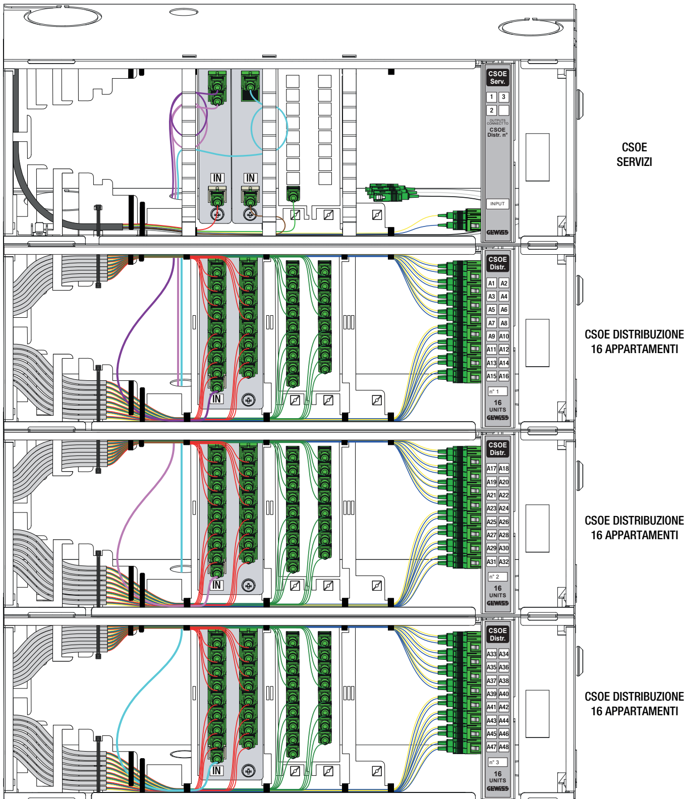
ESEMPIO DI CONFIGURAZIONE FINO A 48 APPARTAMENTI - 1 SERVIZIO
