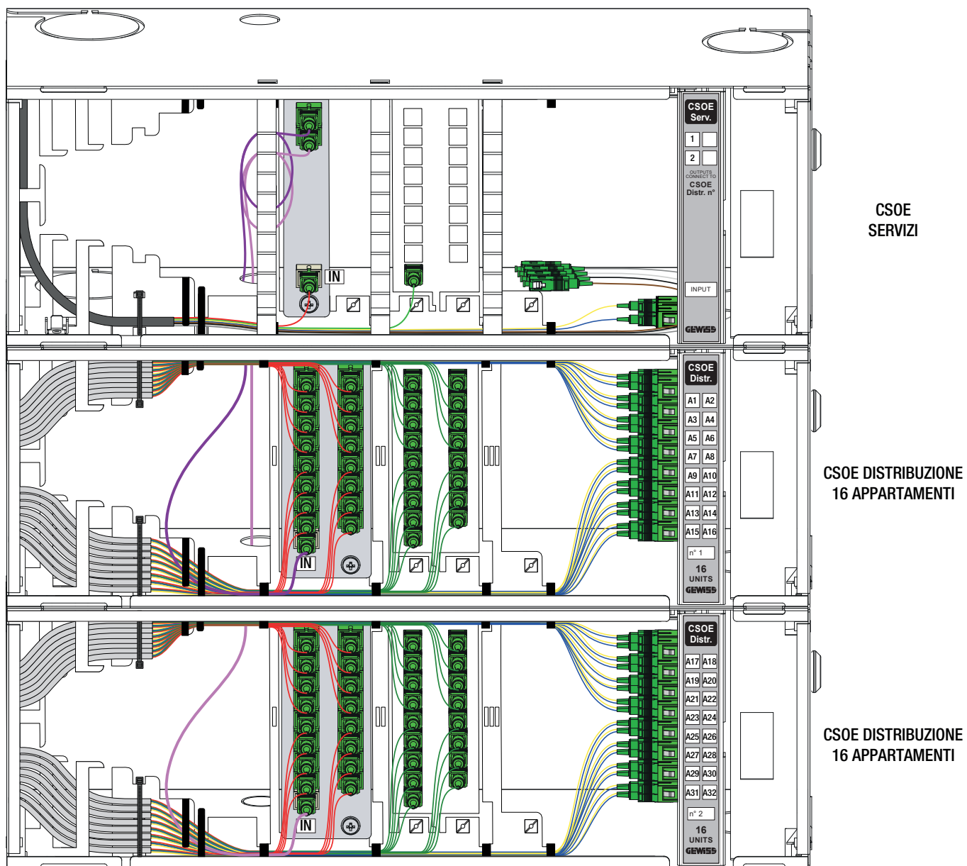
ESEMPIO DI CONFIGURAZIONE FINO A 32 APPARTAMENTI - 1 SERVIZIO
