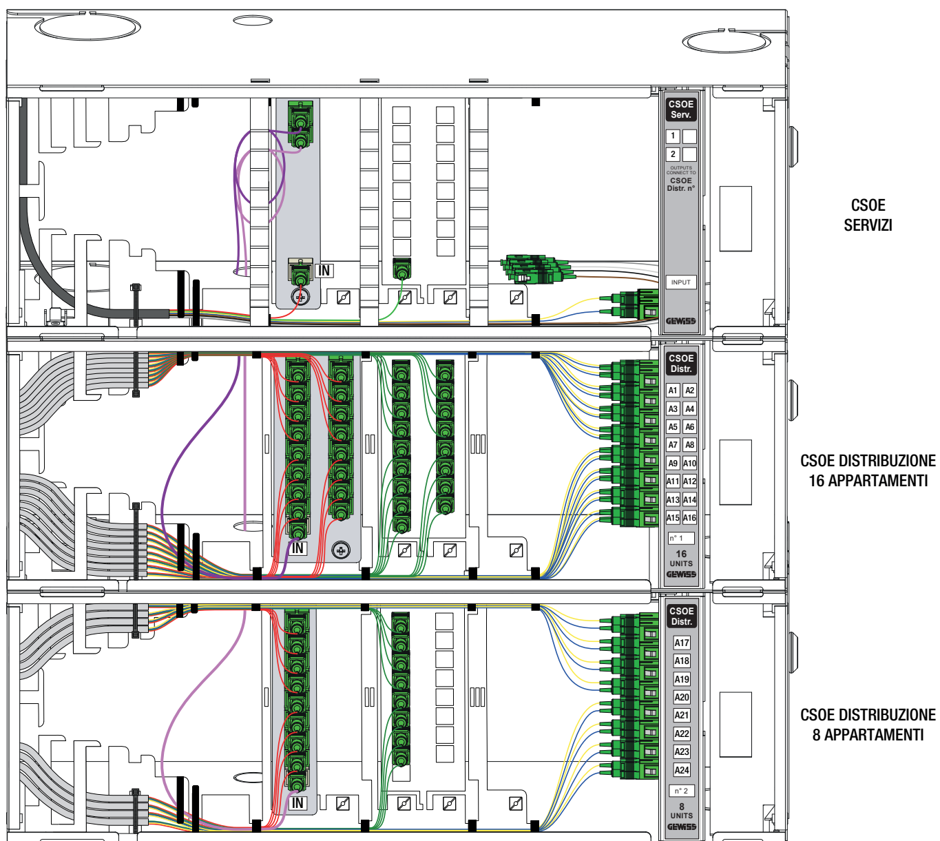
ESEMPIO DI CONFIGURAZIONE FINO A 24 APPARTAMENTI - 1 SERVIZIO
