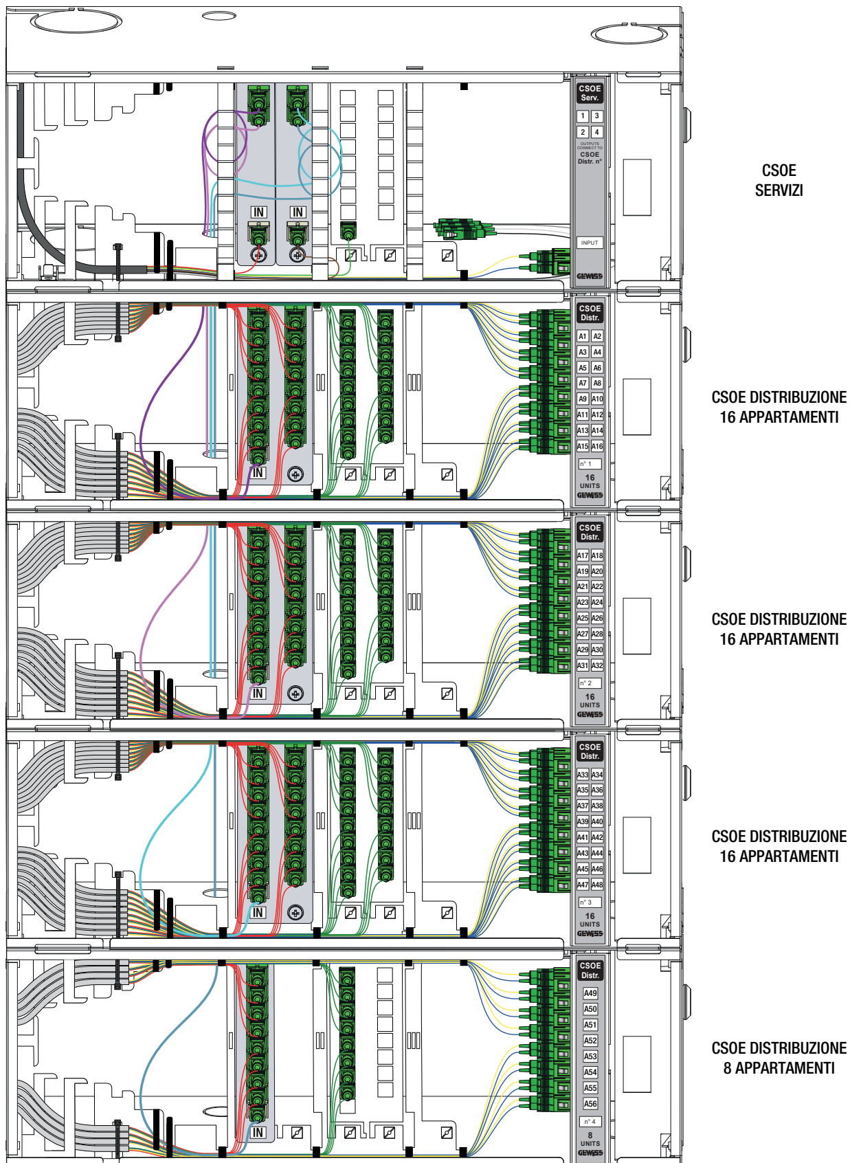
ESEMPIO DI CONFIGURAZIONE FINO A 56 APPARTAMENTI - 1 SERVIZIO
