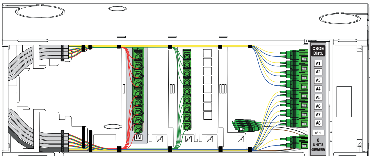
ESEMPIO DI CONFIGURAZIONE FINO A 8 APPARTAMENTI - 1 SERVIZIO
