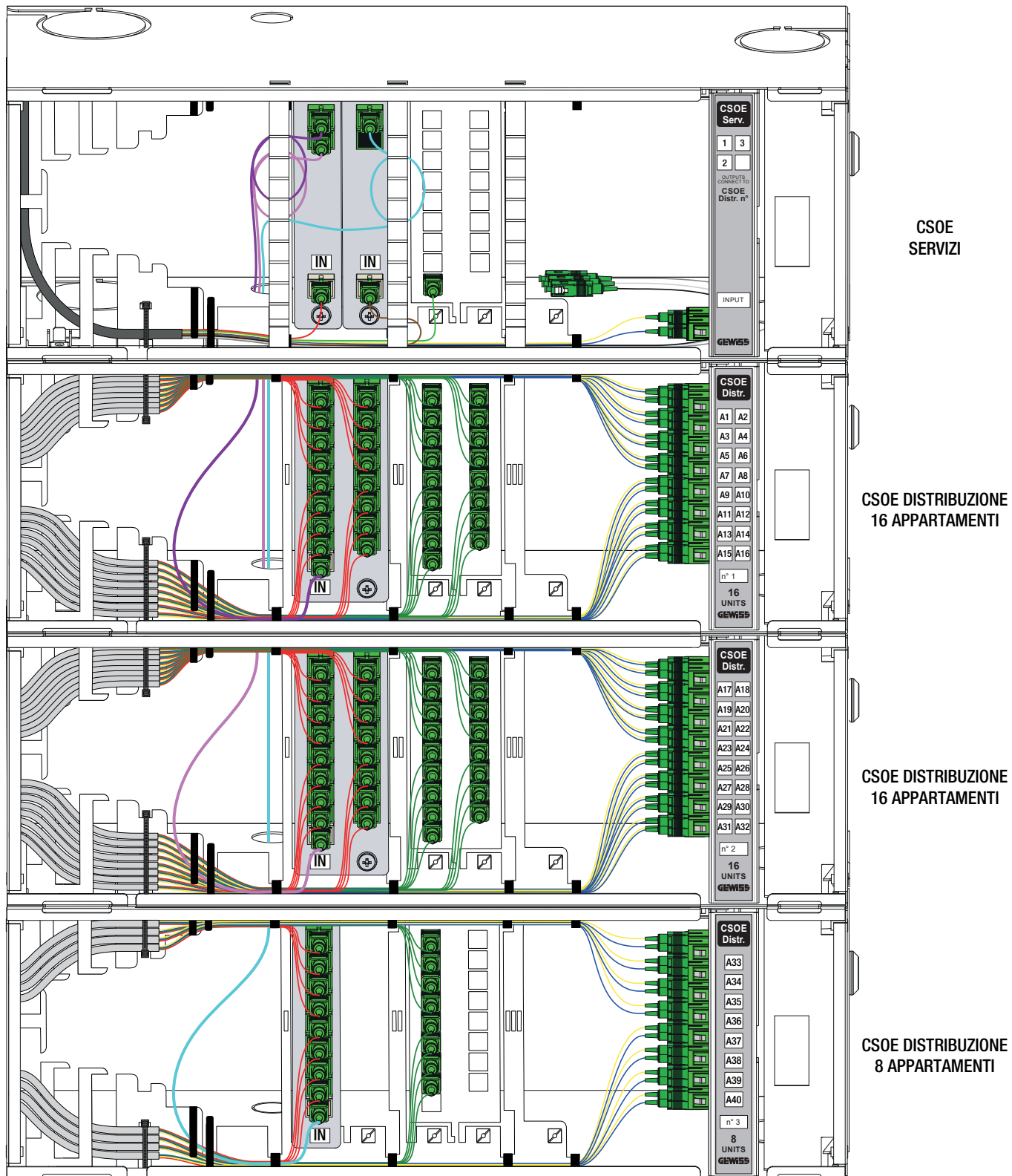
ESEMPIO DI CONFIGURAZIONE FINO A 40 APPARTAMENTI - 1 SERVIZIO
