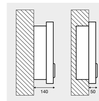
Teilversenkte Montage
