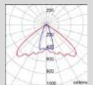
Elliptische Optik
