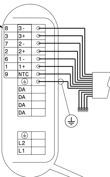
GWP30031 - DALI
