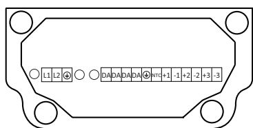
GWP30031 - DALI
