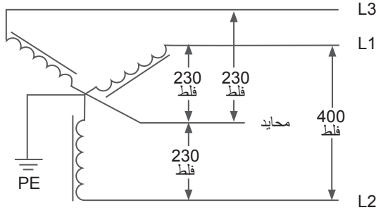
وصلة أسلاك ثلاثية الطور 400 فولت
