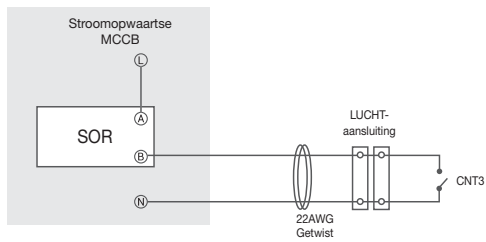
Stuurschakeling
