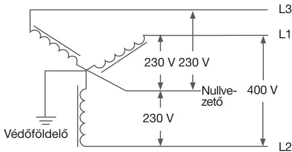
400V-os háromfázisú vezetékes csatlakozás
